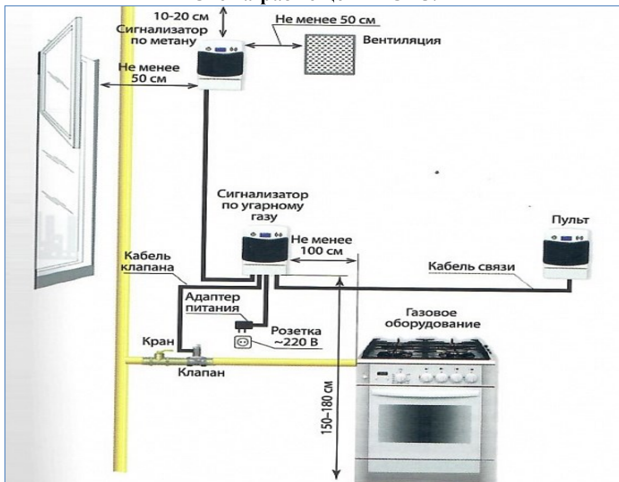
Схема размещения СКЗ.
